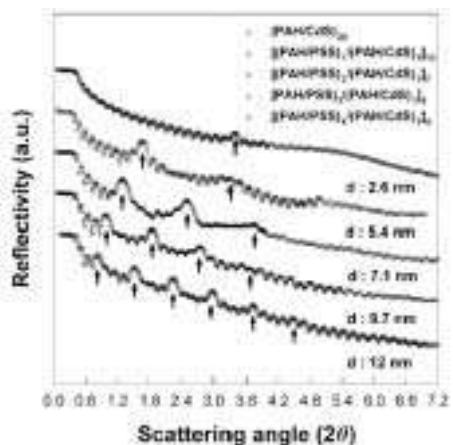
그림 18. Spin SA 방법으로 준비된 [(PAH/PSS) n /(PAH/CdS) 1 ] m ([n+1]×m=20 또는 21) 필름의 X-ray 반사를 곡선. (PAH/PSS) bilayer을 0에서부터 4가지 증가시킬 경우 고분자전해질과 CdS 나노입자 사이의 d-spacing은 2.6 nm에서 12 nm까지 증가된다. 그림에서 나타난 화살표는 각 경우에 대한 Bragg 피크를 나타낸다.
