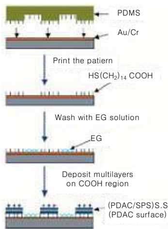
그림 4. 패턴된 기판위에 다층초박막 필름 형성을 위한 공정.
