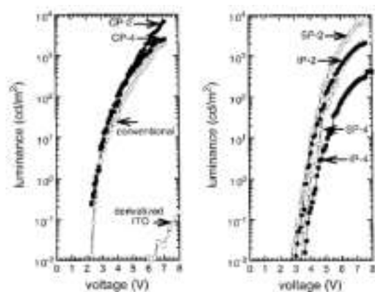
그림 11. 그림 10에서 설명된 소자들의 L(luminance)-V (voltage) 특성.
