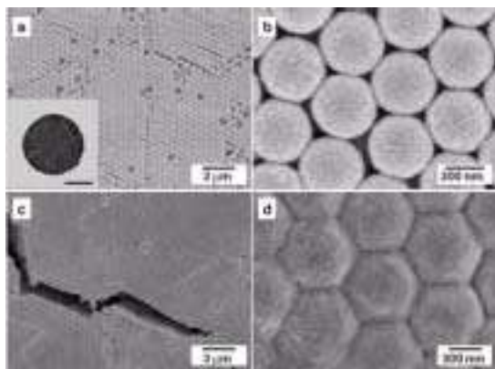
그림 6. (PAH/PSS) 2 /Au/PEI/PSS가 코팅된 폴리스티렌 콜로이드 결정 배열의 SEM 사진 (a,b). (PAH/PSS) 4 /PEO가 코팅된 폴리스티렌 콜로이드 결정배열 사이에 침투된 금 나노입자 (c,d). TEM 사진에서 확인한 폴리스티렌 콜로이드 입자와 금 나노입자 크기는 각각 640 nm와 6 nm으로 확인됨.
