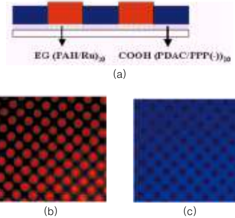
그림 5. (a) COOH 표면 위에 흡착된 (\text{PDAC/PPP})_{10} 과 EG 표면위에 흡착된 (\text{PAH/Ru}(\text{phen})_3^{4-})_{10} 다층초박막 필름. (b) EG 표면위에 흡착된 (\text{PAH/Ru}(\text{phen})_3^{4-})_{10} 필름을 FITC 필터로 찍은 형광현미경 사진 (dot diameter size = 10 μm). (c) COOH 표면위에 흡착된 (\text{PDAC/PPP})_{10} 필름을 DAPI 필터로 찍은 형광현미경 사진.
