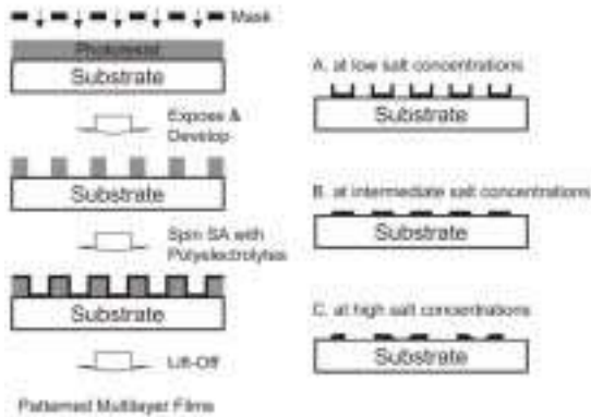
그림 21. Spin SALO (spin SA & Lift-off) 방법을 이용한 다층초박막의 마이크패턴 공정과 이온염 농도에 따른 다양한 패턴 (A~C) 형태.
