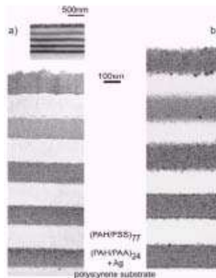
그림 7. 은 나노입자를 함유한 다층박막 필름의 TEM 사진. (a) 다층박막 형성후 silver acetate 용액에 한번 담겼을때의 은 나노입자가 합성된 필름 (ref. Langmuir , 16 , 1354 (2000) 참조). 120±4 nm 두께의 고굴절율 층 (어두운 부분)과 137±6 nm 두께의 저굴절율 층 (밝은 부분)을 구분할 수 있음. (b) 다층초박막을 silver acetate 용액에 5번 담겼을때의 은 나노입자가 합성된 필름. 167±7 nm 두께의 고굴절율 층 (어두운 부분)과 148±9 nm 두께의 저굴절율 층 (밝은 부분)을 보여주고 있음.
