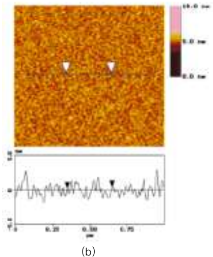
그림 16. (a) spin SA (b) dip SA 방법으로 준비된 (PAH/PSS) 30 다층박막필름의 tapping mode AFM 사진들.
