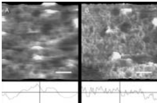
그림 4. (a) Q 조절 없을 때와 (b) Q 조절 있을 때, dekaline (decahydronaphthalene) 속 30% isotactic polystyrene gel 의 AFM 사진. 단위 막대 (scale bar)의 길이는 1 \mu\text{m} 이다.
