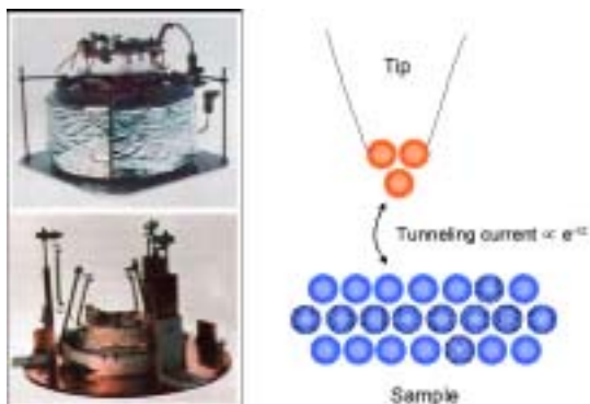
그림 1. (a) 초기 STM의 모습 : 과학계를 놀라게 한 초라한 장치. STM의 제작을 위해서는 터널링 전류를 안정적으로 유지하고 외부 잡음 (noise)을 제거하기 위한 진동 차폐 및 감쇄 (vibration isolation and damping) 시스템과 미세한 움직임을 제어하기 위한 압전 스캐너 (piezo-electric scanner) 기술 등이 뒷받침 되어야한다. (b) STM 측정 시 터널링 전류는 팁과 시료 사이의 거리, z 가 증가하면 지수적으로 급격히 감소한다.
