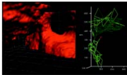
그림 13. (왼쪽) Agar 그물구조 (network)의 열잡음 (thermal noise) 사진. (오른쪽) 광 에너지 우물에 포획된 입자의 이동경로 (trajectory). 점탄성 (viscoelasticity)에 관한 정보를 얻을 수 있으며, 경로의 시작점은 붉은 점으로 끝점은 붉은 화살표로 나타내었다.
