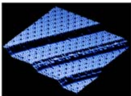
그림 2. Si(111)- 7 \times 7 재배열 (reconstruction) 표면에 형성된 원자 계단의 STM 사진.
