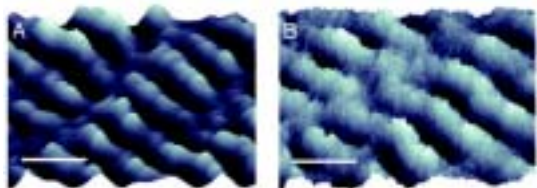
그림 12. PHB/V [poly(hydroxybutyrate-co-hydroxyvalerate)] 구형체 (spherulite)의 광학적 주름 (optical banding)에 대한 SNOM 사진. (a) 일반적인 방법을 사용하여 20분에 걸쳐 얻은 사진. (b) 고속 공명 스캔 방식을 사용하여 8.3 ms 만에 얻은 사진. 크기막대 (Scale bars)는 1 \mu\text{m} 를 나타낸다.
