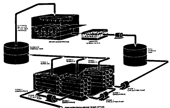
그림 8. 섬유호제 처리를 위한 한외여과 분리 공정.
