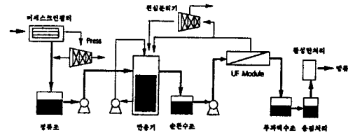
그림 10. 한외여과막을 이용한 분별처리 시스템 공정도.
