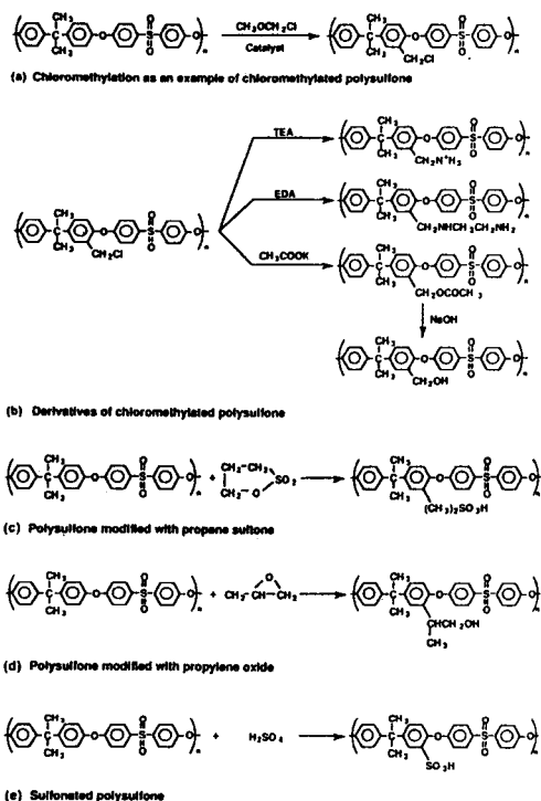
그림 4. 폴리설폰 고분자의 개질방법.
