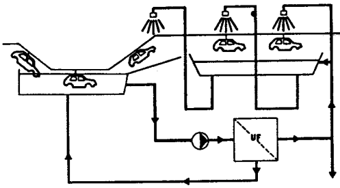
그림 6. 한외여과막을 이용한 전착도료 회수 공정 개념도.
