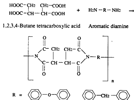
그림 3. 폴리이미드의 합성법.
