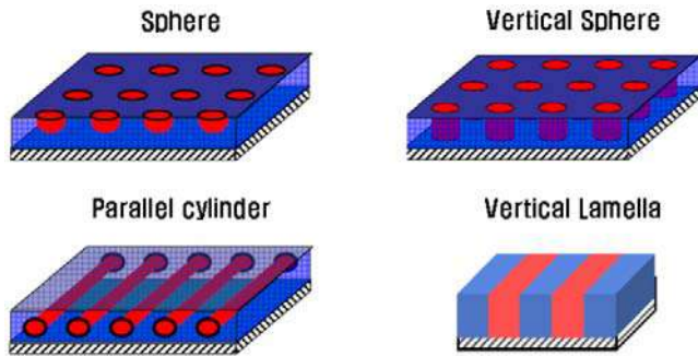
그림 2. 블록 공중합체 나노구조체의 배향.
