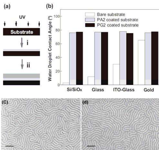
그림 10. (a) 광경화형 랜덤 공중합체를 사용한 중성 표면 제작 과정의 모식도. (b) 다양한 기판에서 광경화 반응 후의 물방울 접촉각. (c) 그리고 (d) 실리콘 기판과 금 코팅 기판 위에서의 수직 배향된 리멜라형 블록 공중합체 나노구조체 SEM 사진들.
