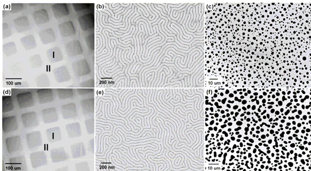
그림 11. (a) 그리고 (c) 비닐 그룹을 가지는 광경화형 랜덤 공중합체를 사용한 배향 패터닝 구조의 SEM 사진들. (b), (c), (e) 그리고 (f) SEM 사진 (a)와 (c)에서의 영역 I과 II의 확대 SEM 사진.
