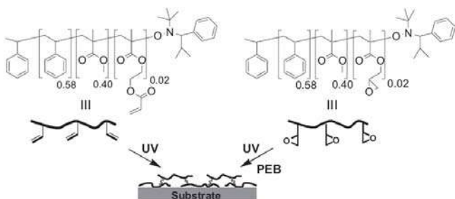
그림 9. 광경화형 랜덤 공중합체를 사용한 중성 표면 제작 기술.
