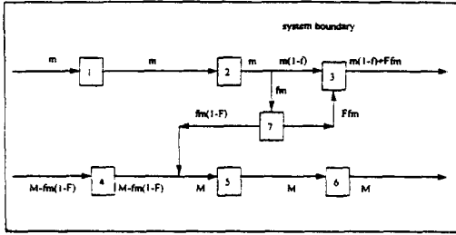
그림 11. Schematic diagram showing open loop recycling.
