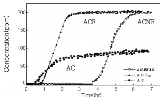
그림 11. Adsorption behaviors of toluene on the CNFs. 21,22
