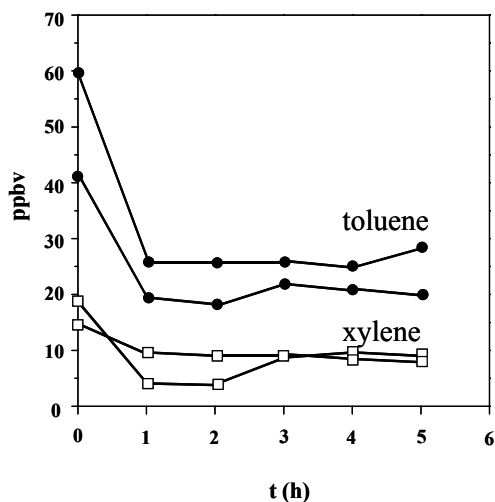
그림 4. \text{TiO}_2 광촉매 반응을 이용한 톨루엔과 크실렌의 분해. 18
