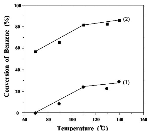
그림 3. 열(1)과 열과 TiO 2 광촉매 반응 (2)을 이용한 벤젠의 분해. 17)
